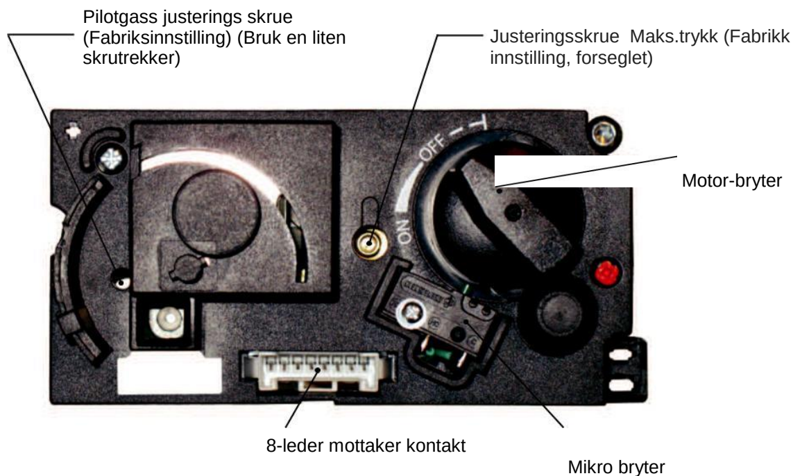
Figur 4: Gassreguleringsblokk
