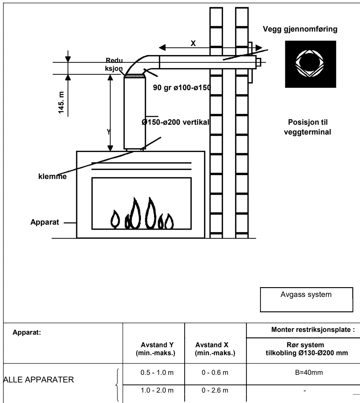
Figur 11: Horisontal vegg gjennomføring ALLE STØRRELSER INKLUDERER LENGDEN AV TAK ELLER VEGG GJENNOMFØRINGEN
