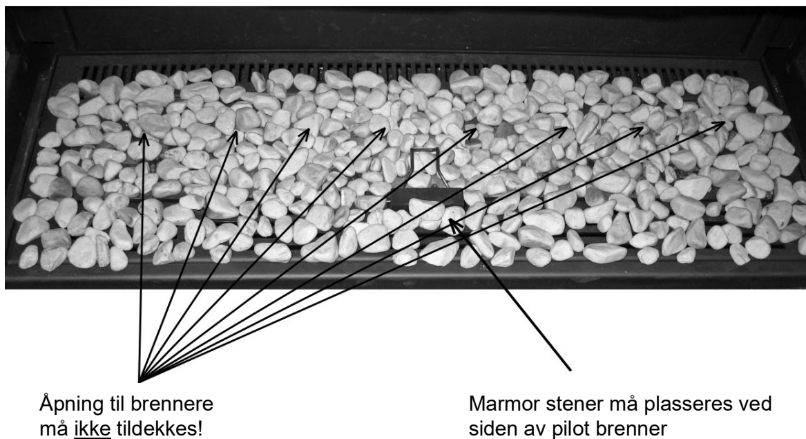
Figur 37: Plassering marmor steiner, Posisjon natur gass og propan/butan brenner
