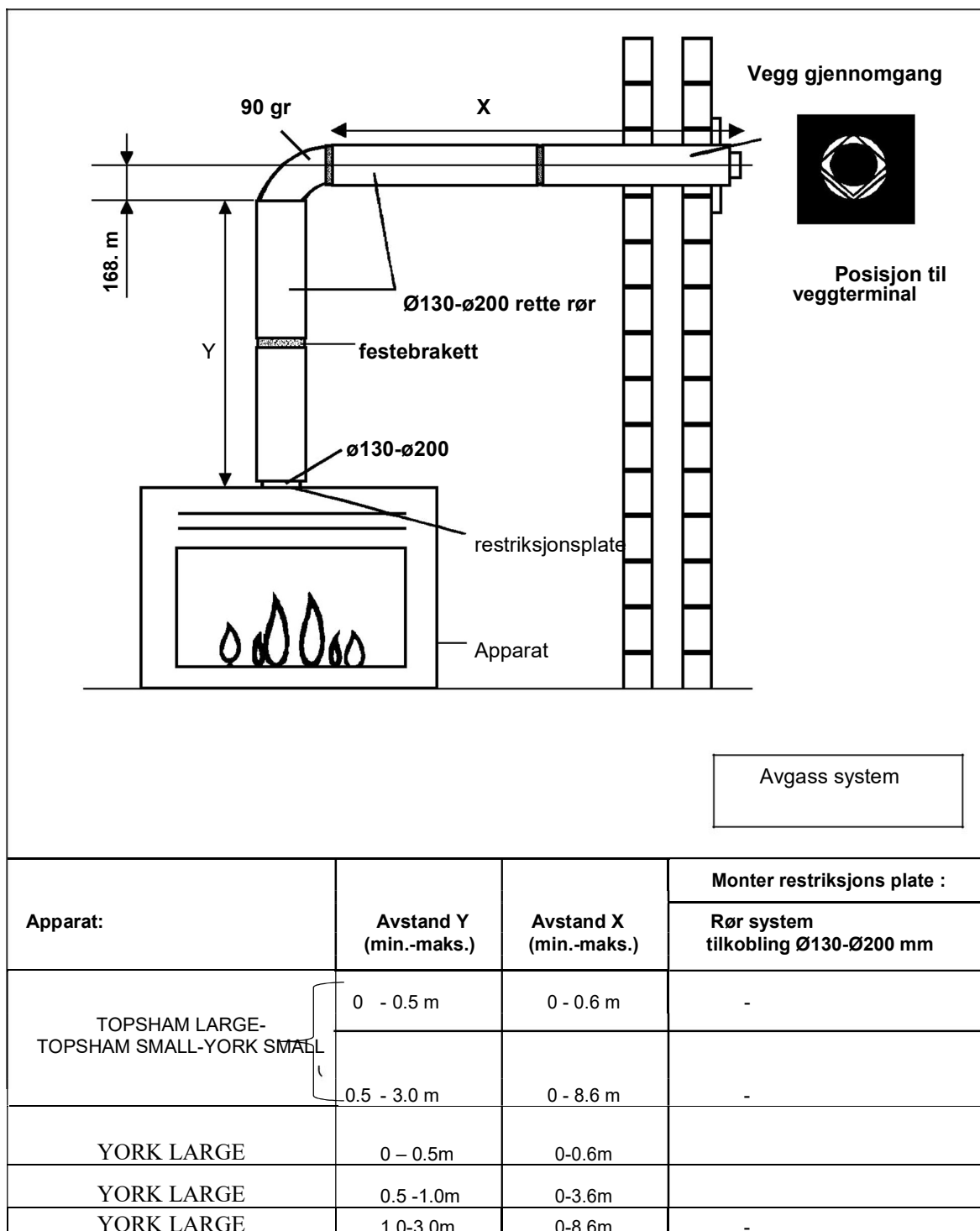
Figur 14: Horisontal vegg gjennomføring
